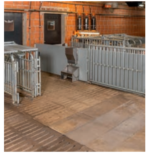
Case d'intégration séparée pour les jeunes truies afin de les inclure facilement dans des bâtiments existants ; utilisation possible en supplément en tant que case pour malades
