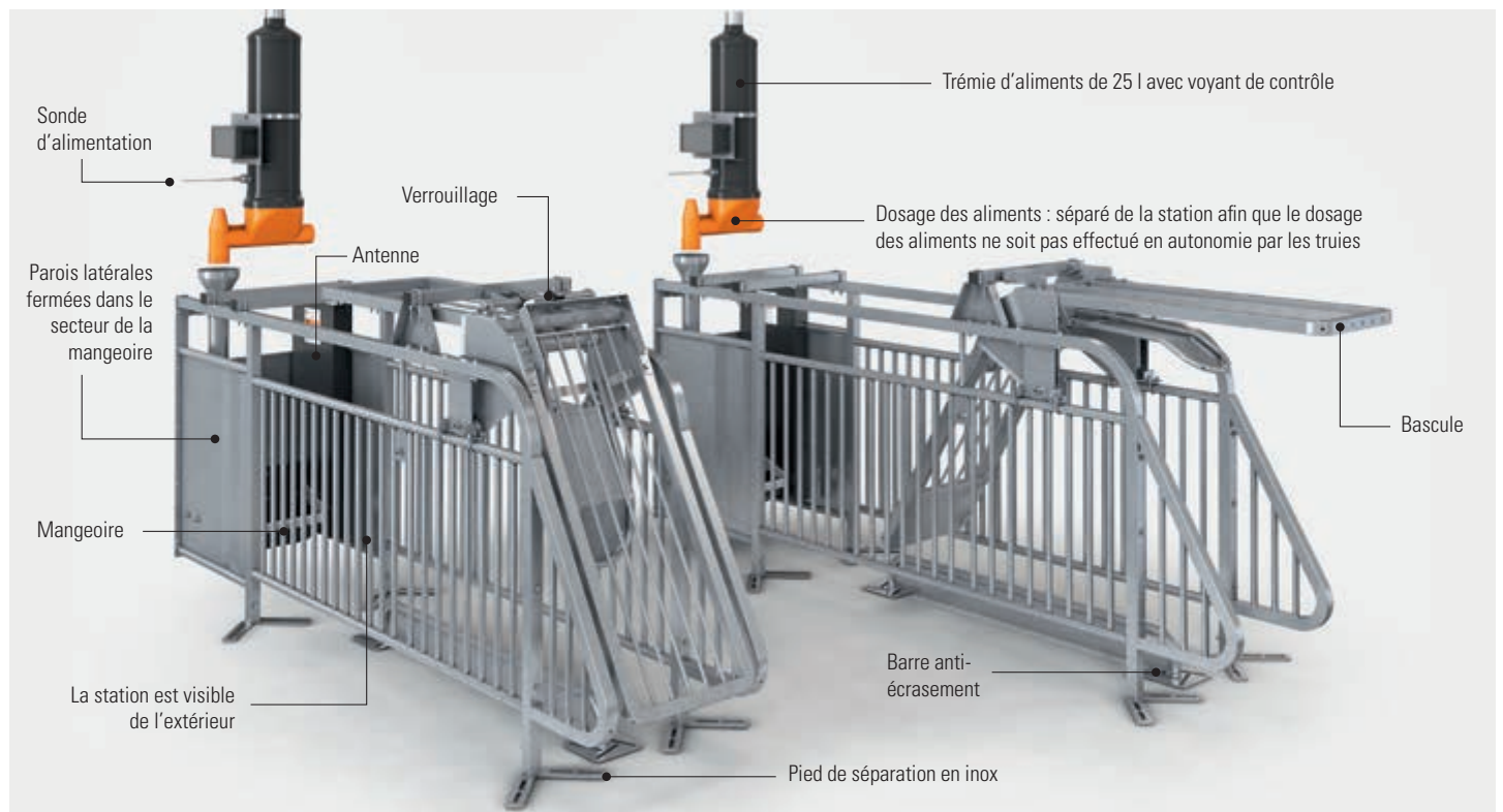
Une barre anti-écrasement empêche que la truie ne reste trop longtemps dans la station
